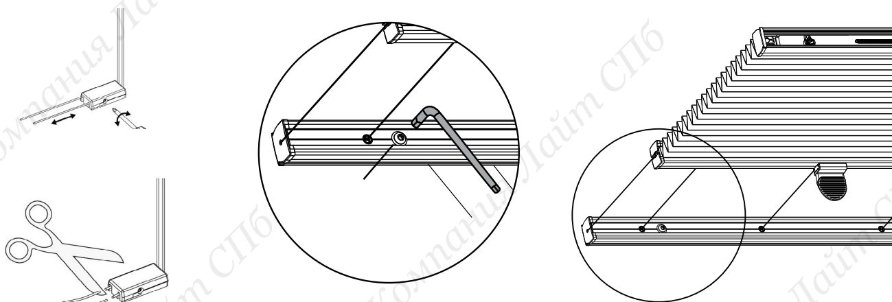
Регулировка натяжения троса в моделях P3xxx.
