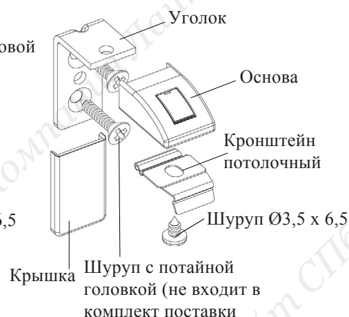
схема сборки стенового закрытого кронштейна
